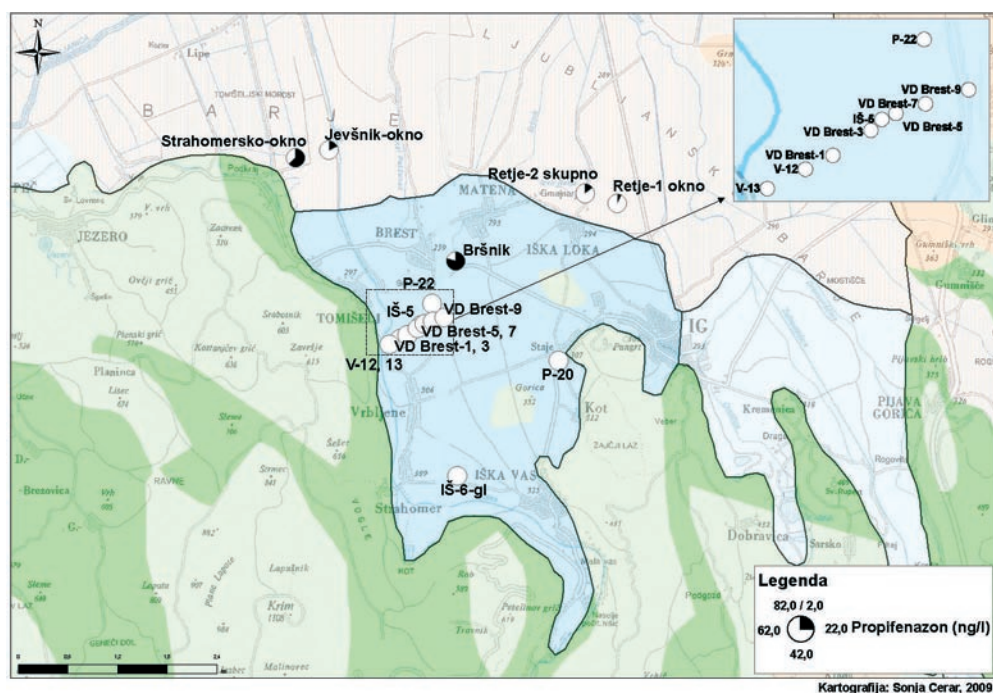
Slika 8. Propiphenazon v vrtinah in izviri na Ljubljanskem barju
