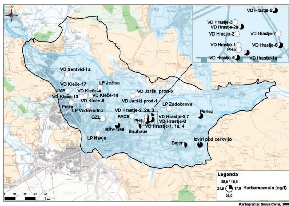
Slika 6. Karbamazepin v vrtinah in izvirih na Ljubljanskem polju
