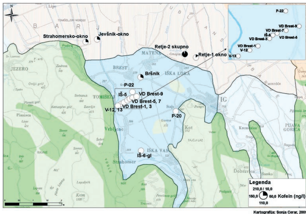
Slika 7. Kofein v vrtinah in izviri na Ljubljanskem barju
