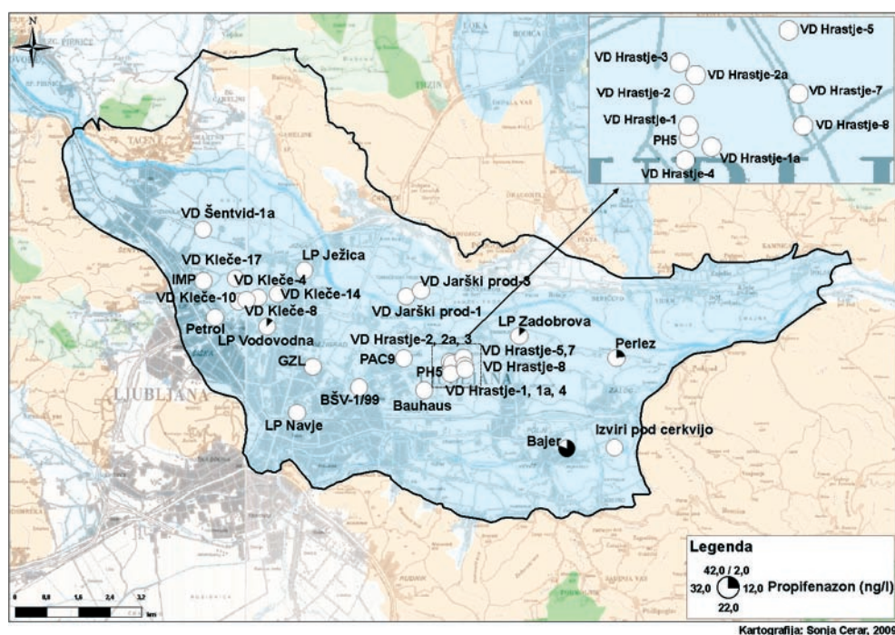
Slika 5. Propifenazon v vrtinah in izvirih na Ljubljanskem polju
